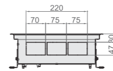
Вид с торца Qtherm 310 с F-образным бортом.
