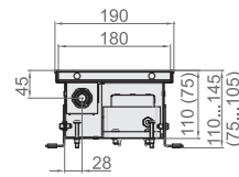
Разрез Qtherm 190 с U-образным бортом.
