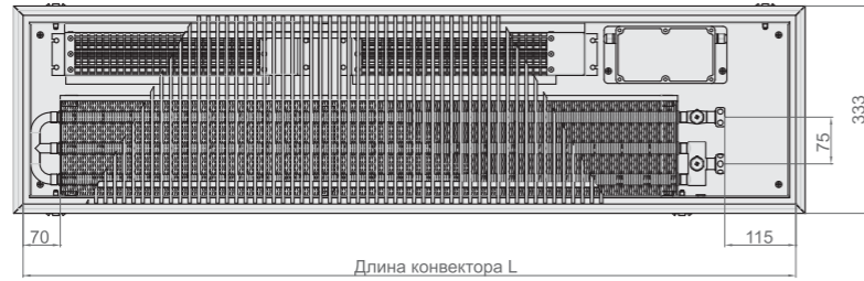
Вид сверху конвектора Qtherm 310 с роликовой решеткой, с F-образным бортом.
