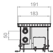
Разрез Qtherm 190 с U-образным бортом.
