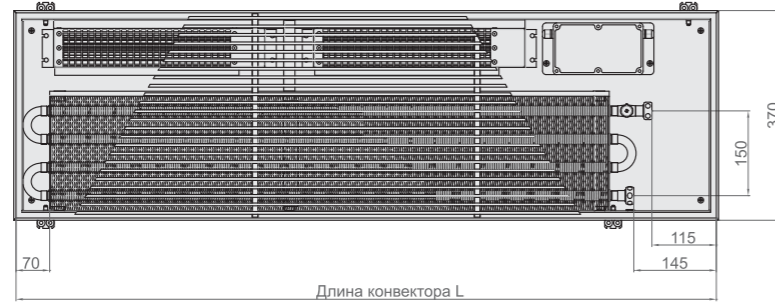
Вид сверху конвектора Qtherm 370 с линейной решеткой, с U-образным бортом.
