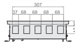
Вид с торца Qtherm 370 с U-образным бортом.
