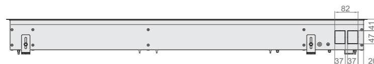
Вид сбоку конвектора Qtherm 250 с F-образным бортом.
