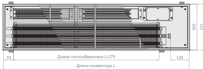
Вид сверху конвектора Qtherm 250 с роликовой решеткой, с U-образным бортом.
