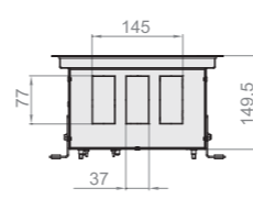
Вид с торца Qtherm 250 с F-образным бортом.
