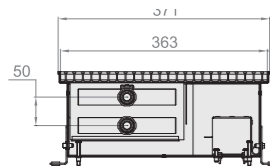
Разрез Qtherm 250 с F-образным бортом.
