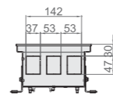
Вид с торца Qtherm 190 с U-образным бортом.
