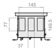
Вид с торца Qtherm 190 с U-образным бортом.
