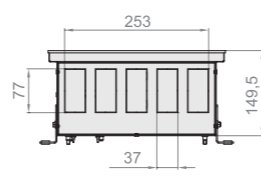
Вид с торца Qtherm 250 с U-образным бортом.
