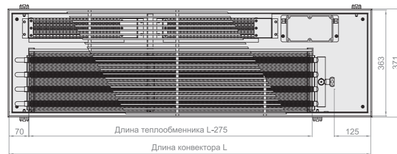
Вид сверху конвектора Qtherm 250 с роликовой решеткой, с F-образным бортом.
