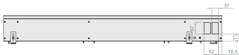
Вид сбоку конвектора Qtherm 250 с U-образным бортом.
