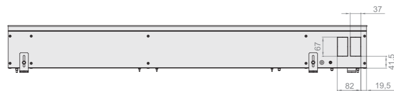
Вид сбоку конвектора Qtherm 190 с U-образным бортом.
