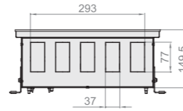
Вид с торца Qtherm 250 с F-образным бортом.
